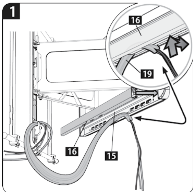
1. 下側のカバーは、図のように壁掛金具 [15] の下側の溝にカバーの下側をはめてからカバーの上側を押し込むようにはめます。
