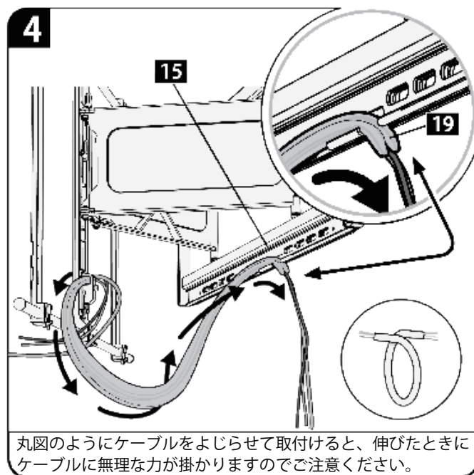
4. 図のように、壁掛金具 [15] を一杯に引き出した時にも余裕が出るようにケーブルを弛ませて、ケーブルカバーを壁掛金具 [15] の溝にかけるように通します。
