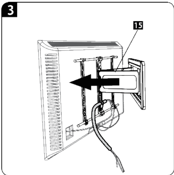
3. 図のように、壁掛金具 [15] のアームをいっぱい引き出します。
