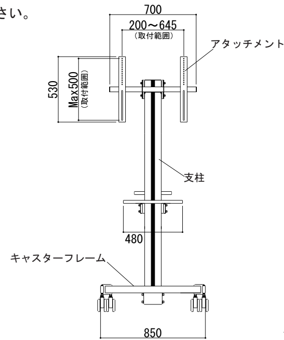
寸法図
