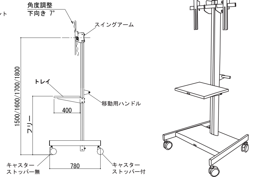
完成図
