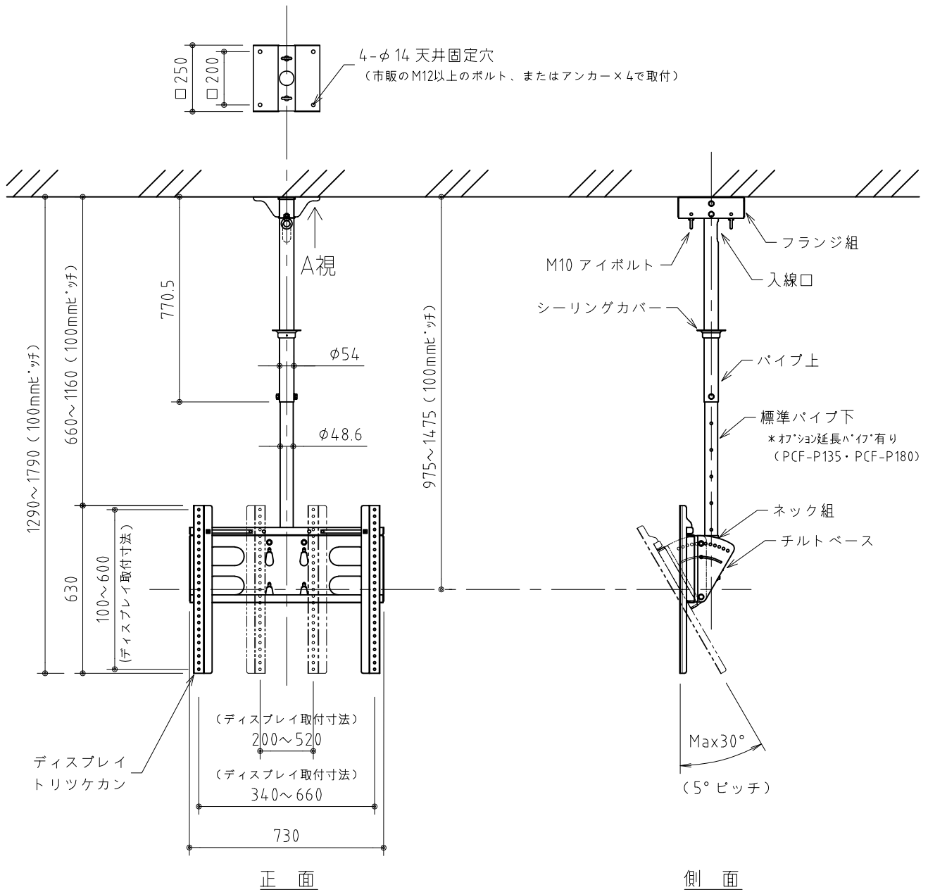
【A矢视图】フランジ取付部
