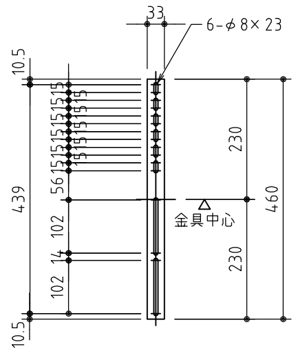
アタッチメント穴位置図 S=1/10
