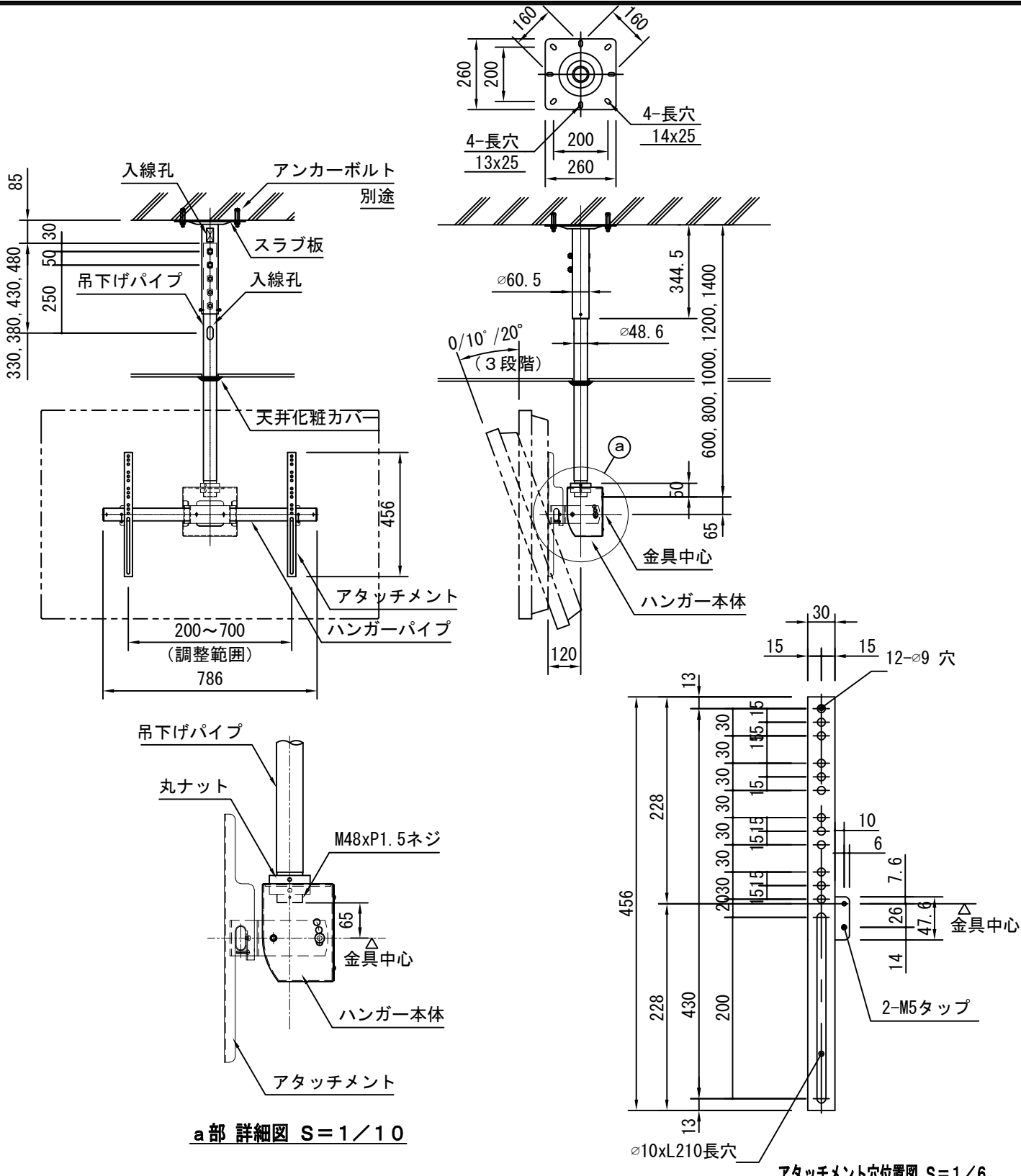
アタッチメント穴位置図 S=1/6
