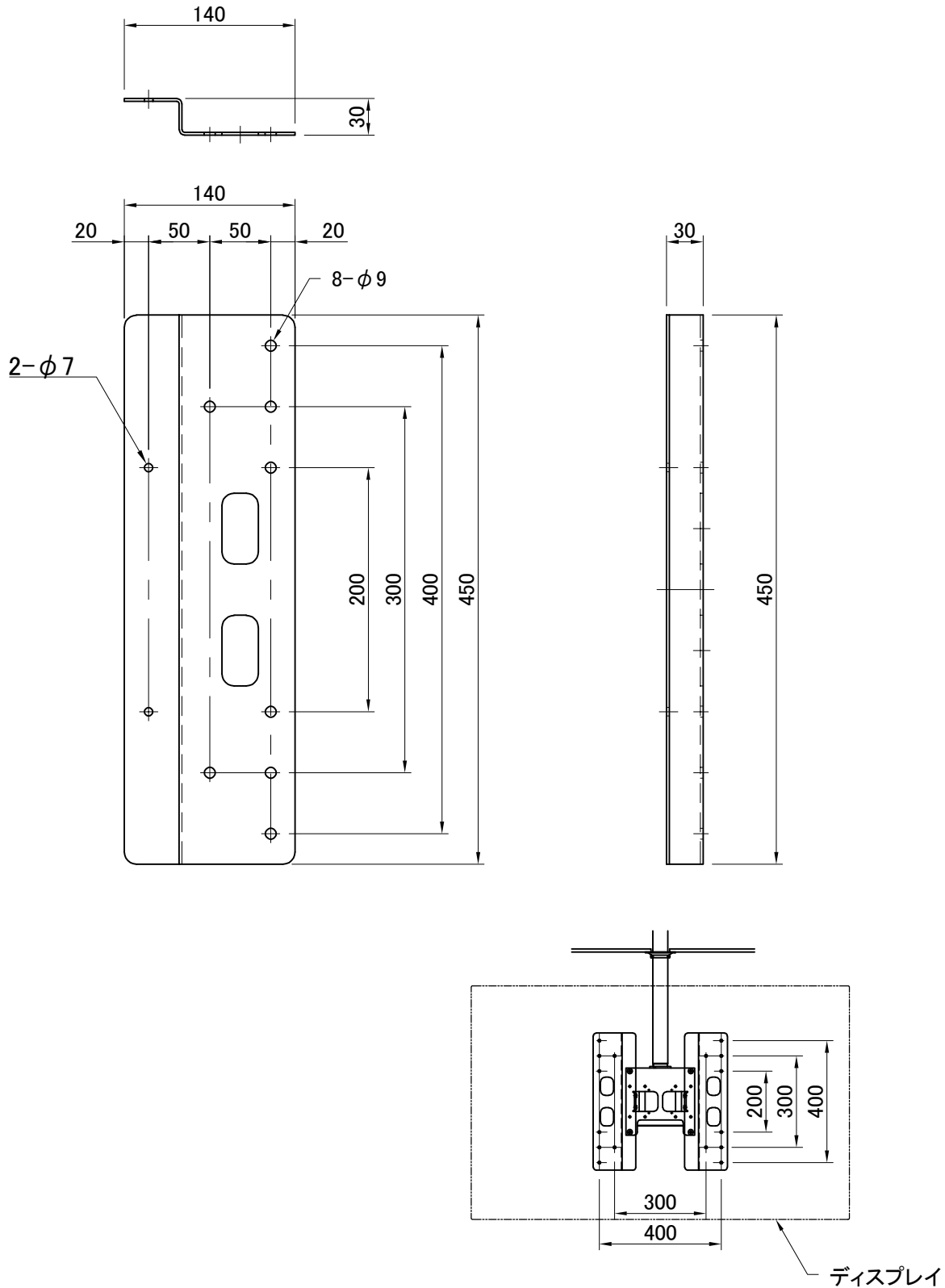
KDHV 組込図 S=1/20
