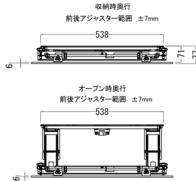
収納時奥行 前後アジャスター範囲 ±7mm
