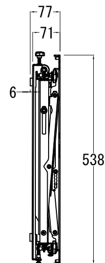
収納時奥行 前後アジャスター範囲 ±7mm
