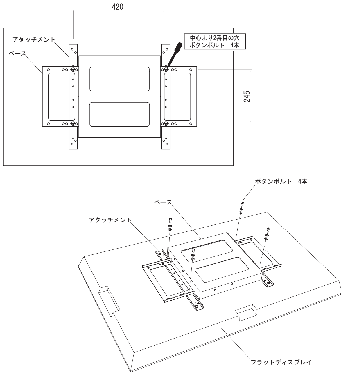
本体ベース部取り付け図
