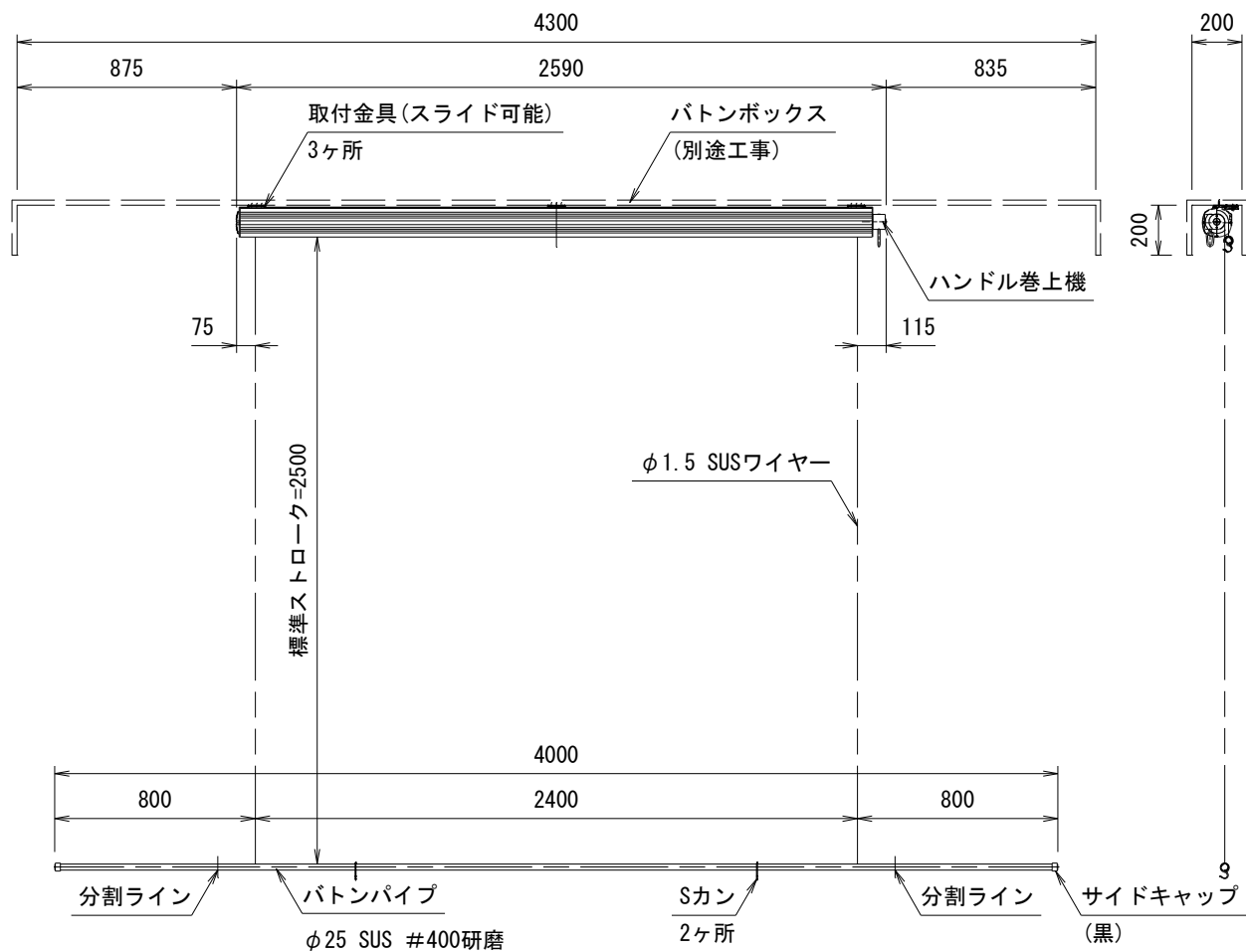
外観図 S=1/30
