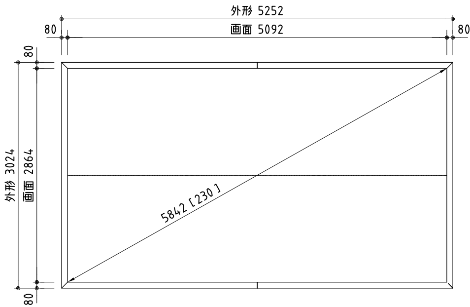
外観図 S=1/50
