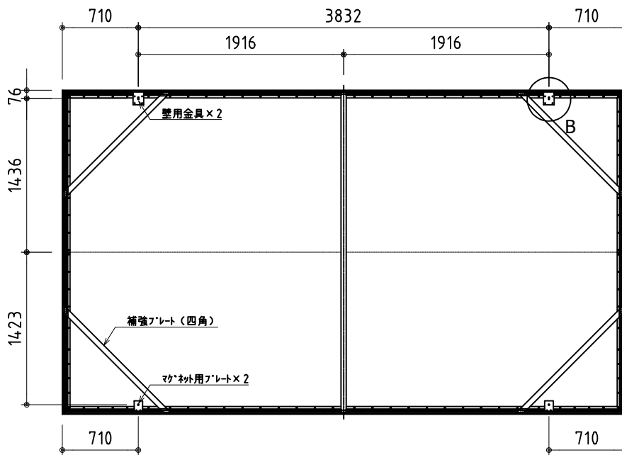
外観図(背面) S=1/50
