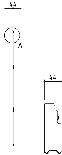
A部 詳細(1:5)
