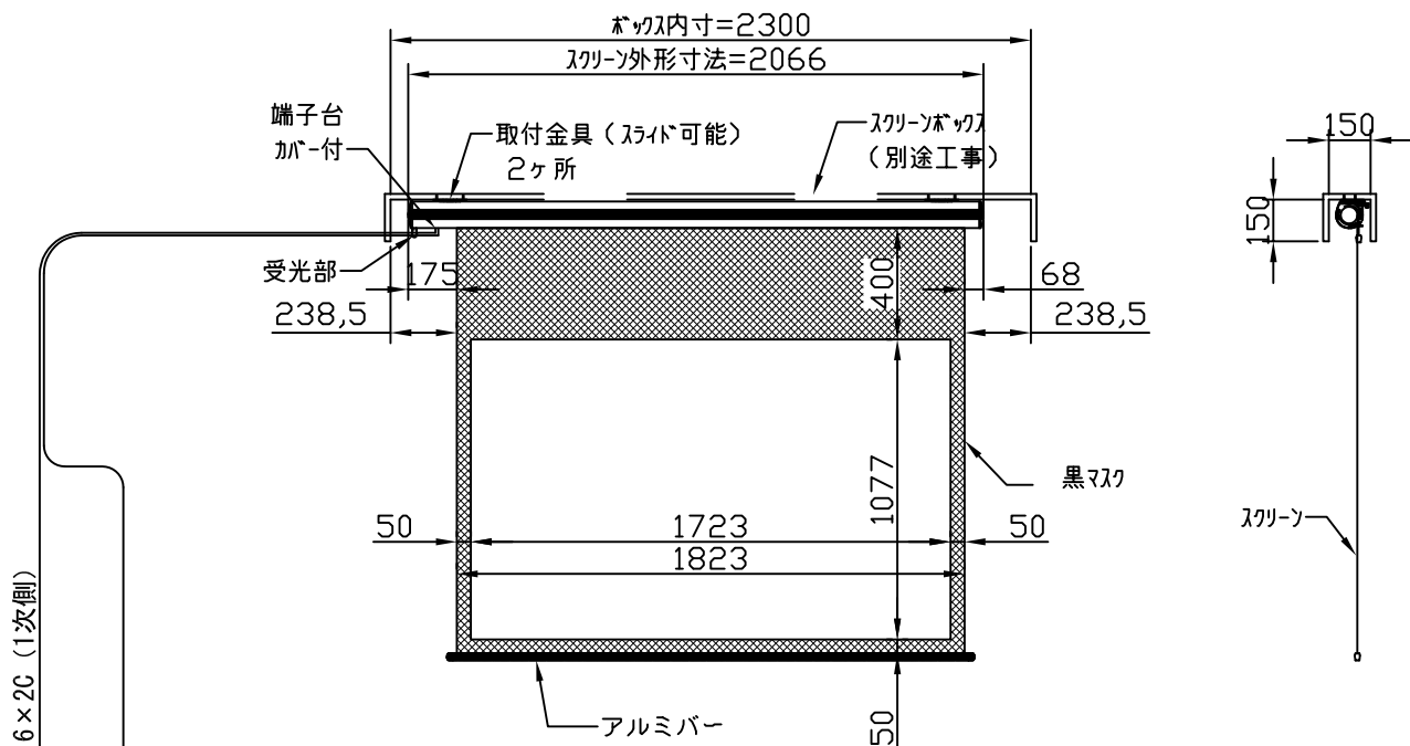
外観図 1/30
