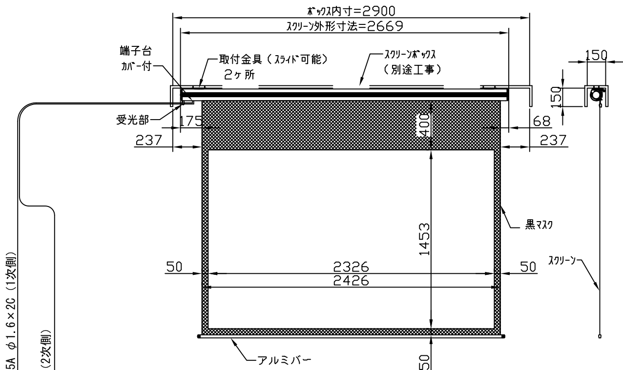
外観図 1/30
