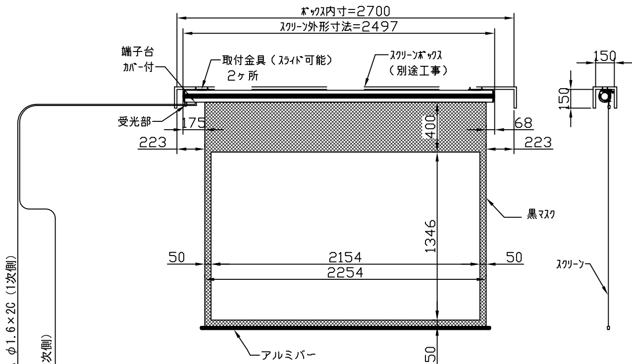
外観図 1/30
