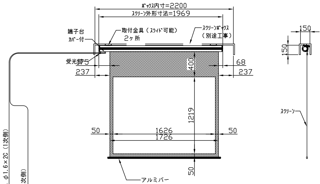
外観図 1/30
