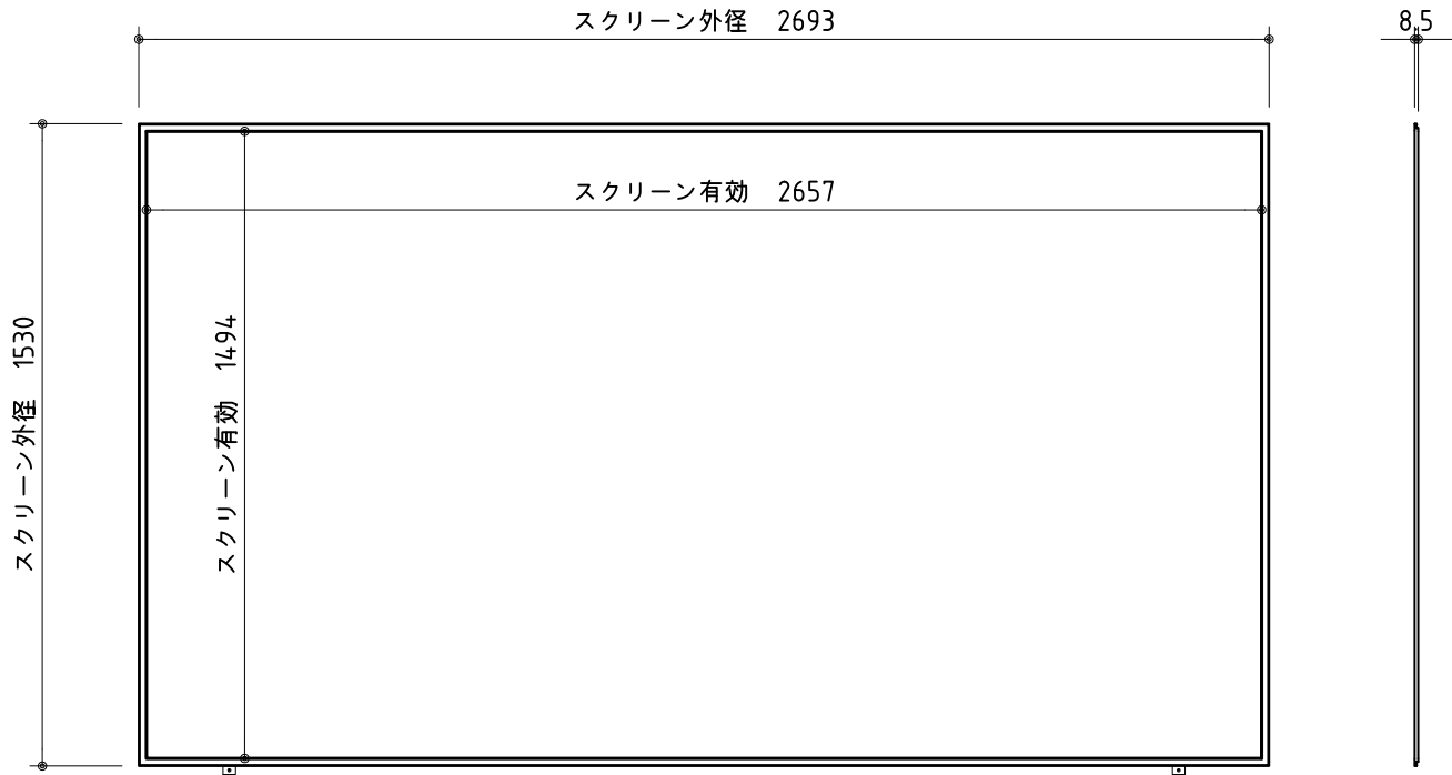
外観図 S=1/20
