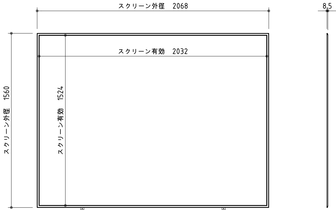
外観図 S=1/20
