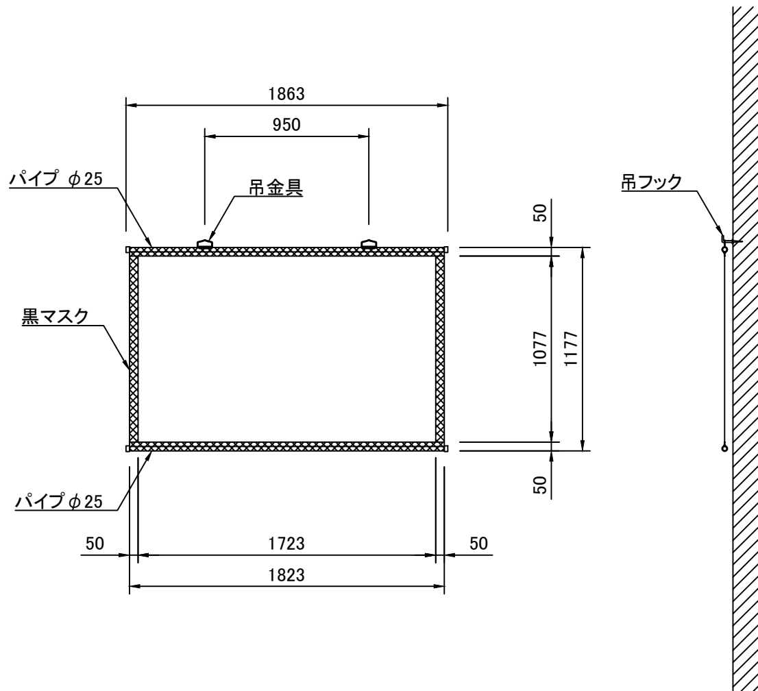
外観図 S=1/30
