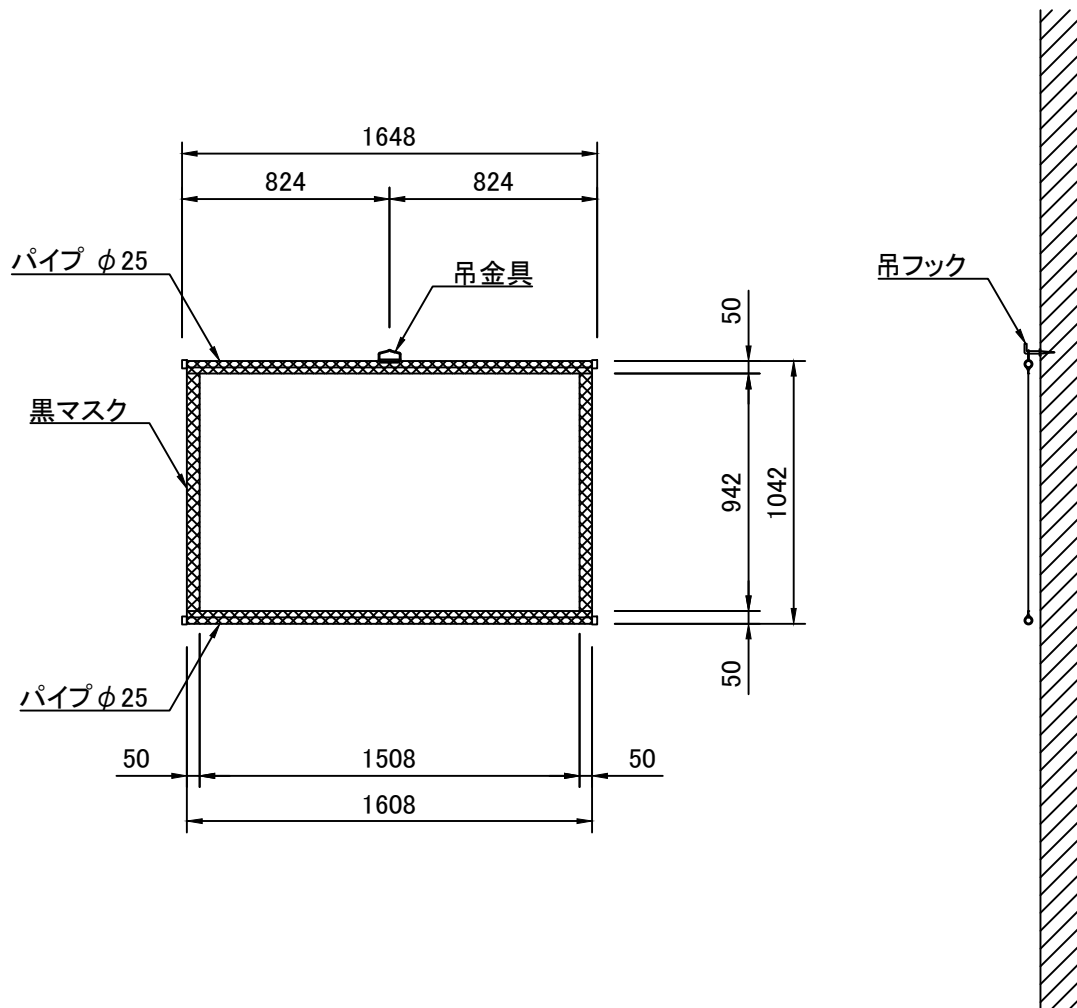
外観図 S=1/30
