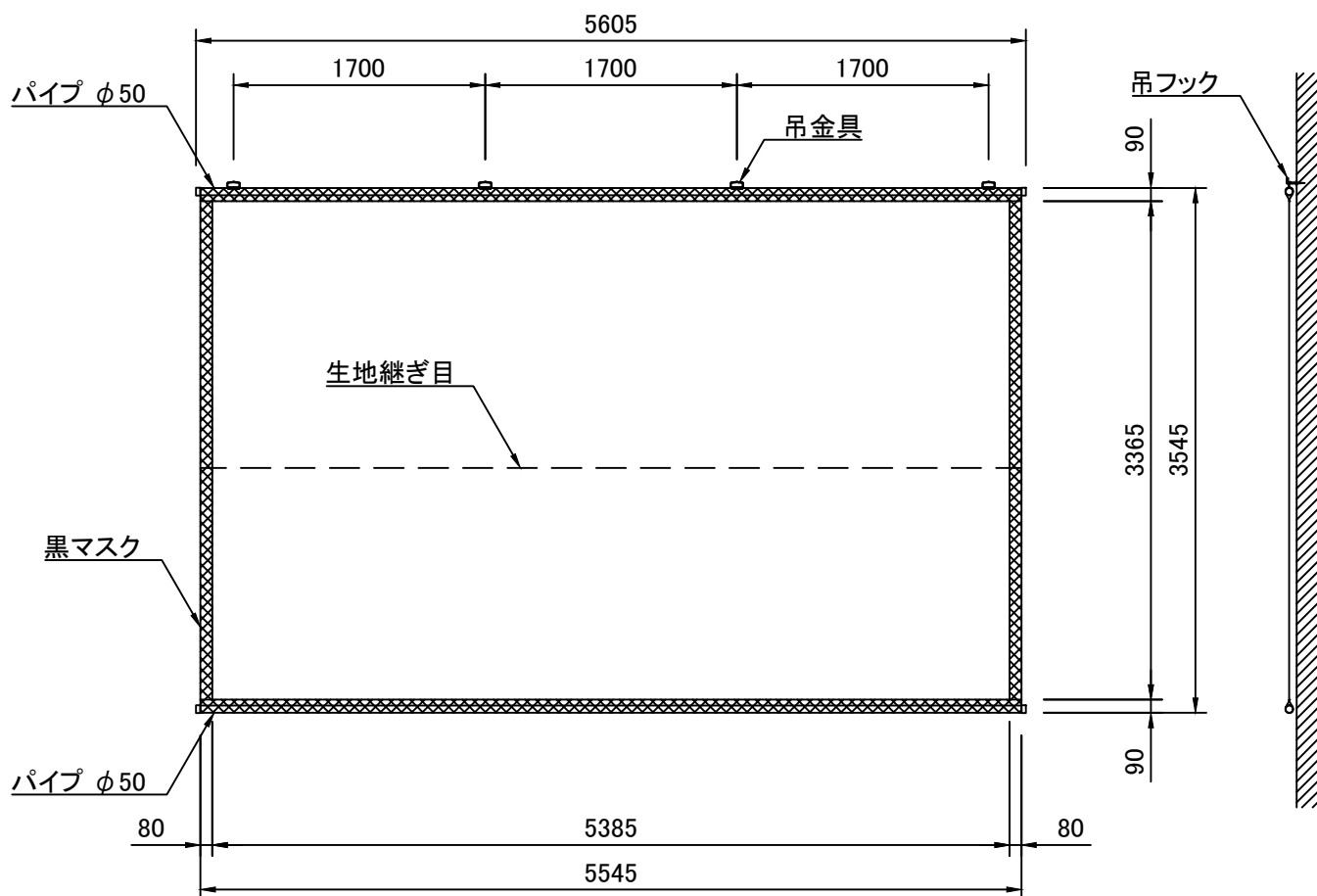
外観図 S=1/50
