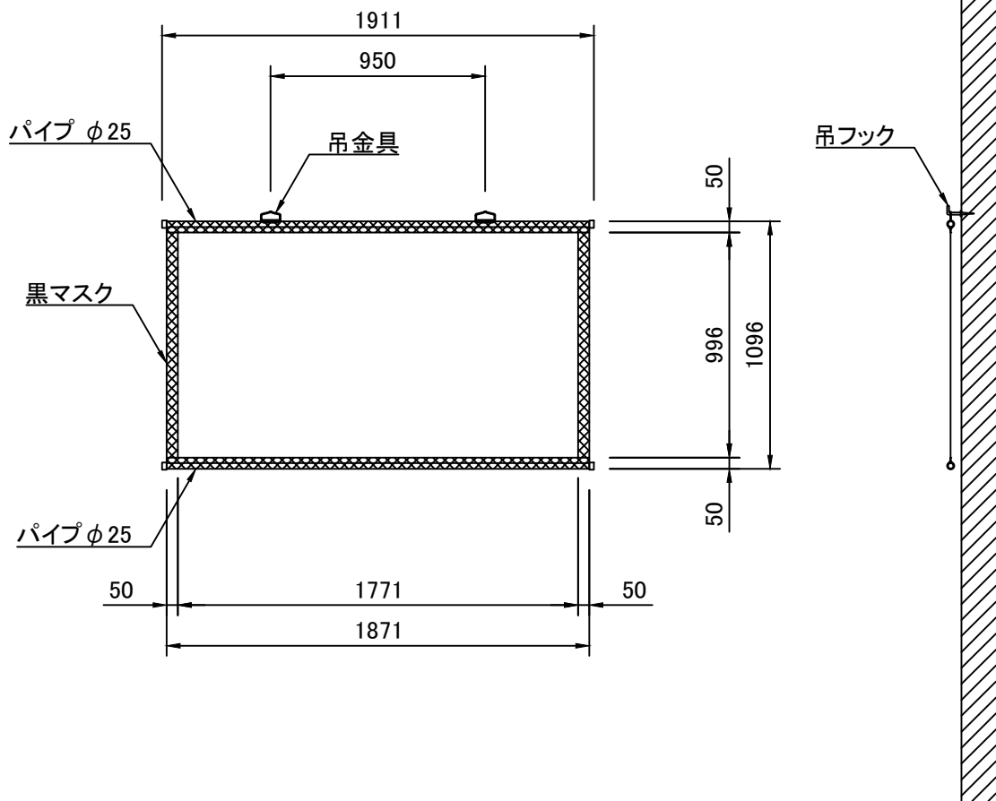
外観図 S=1/30
