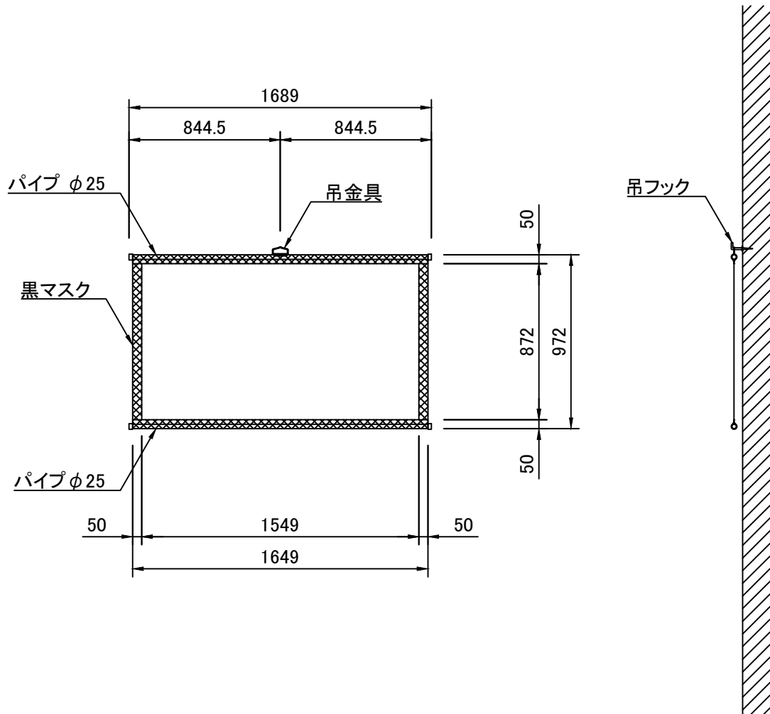
外観図 S=1/30
