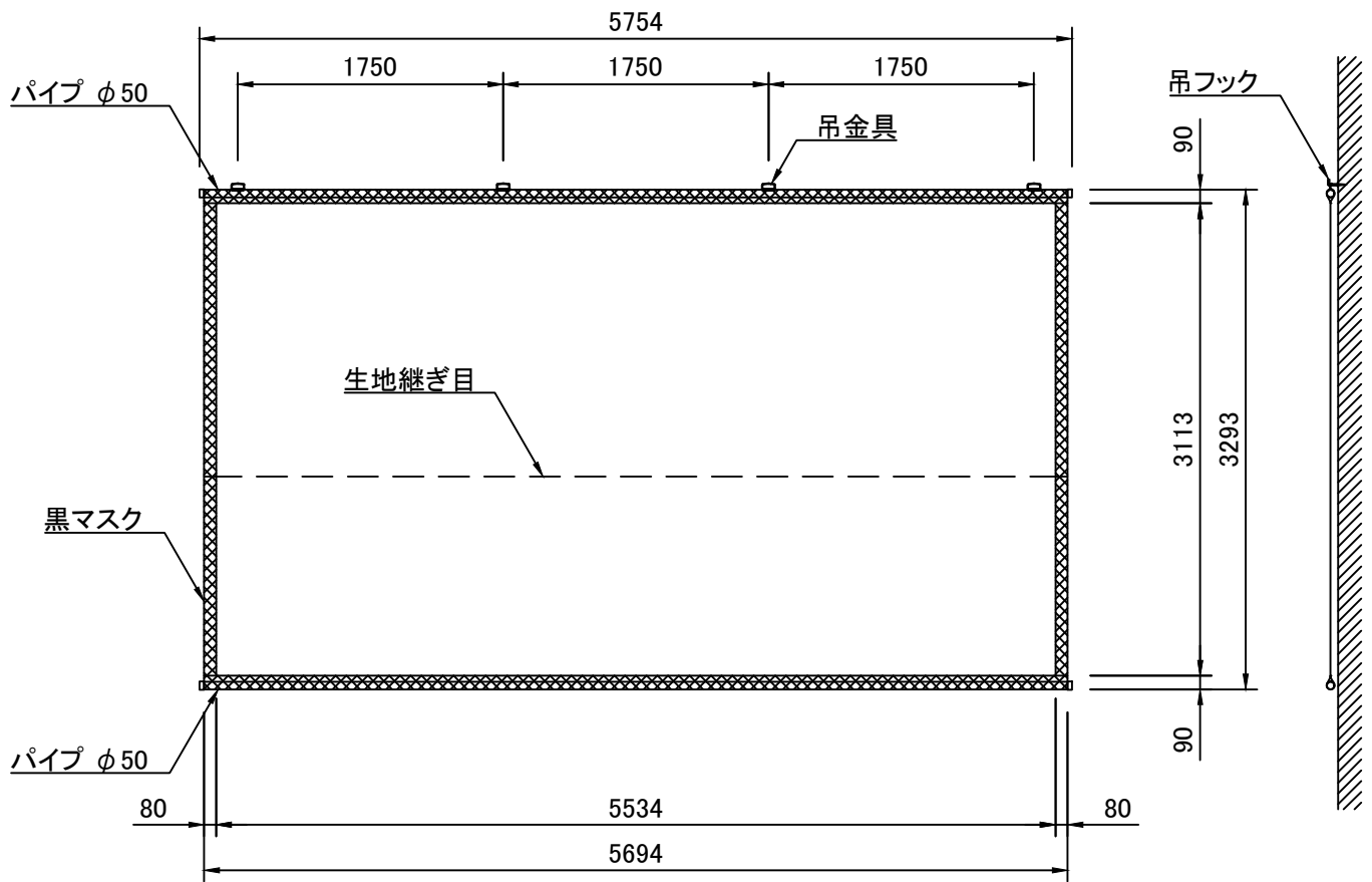
外観図 S=1/50
