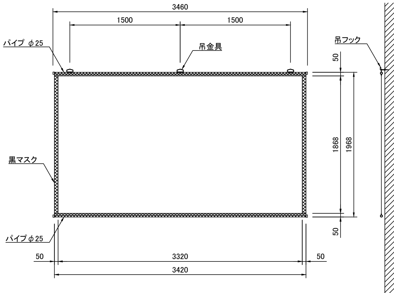
外観図 S=1/30
