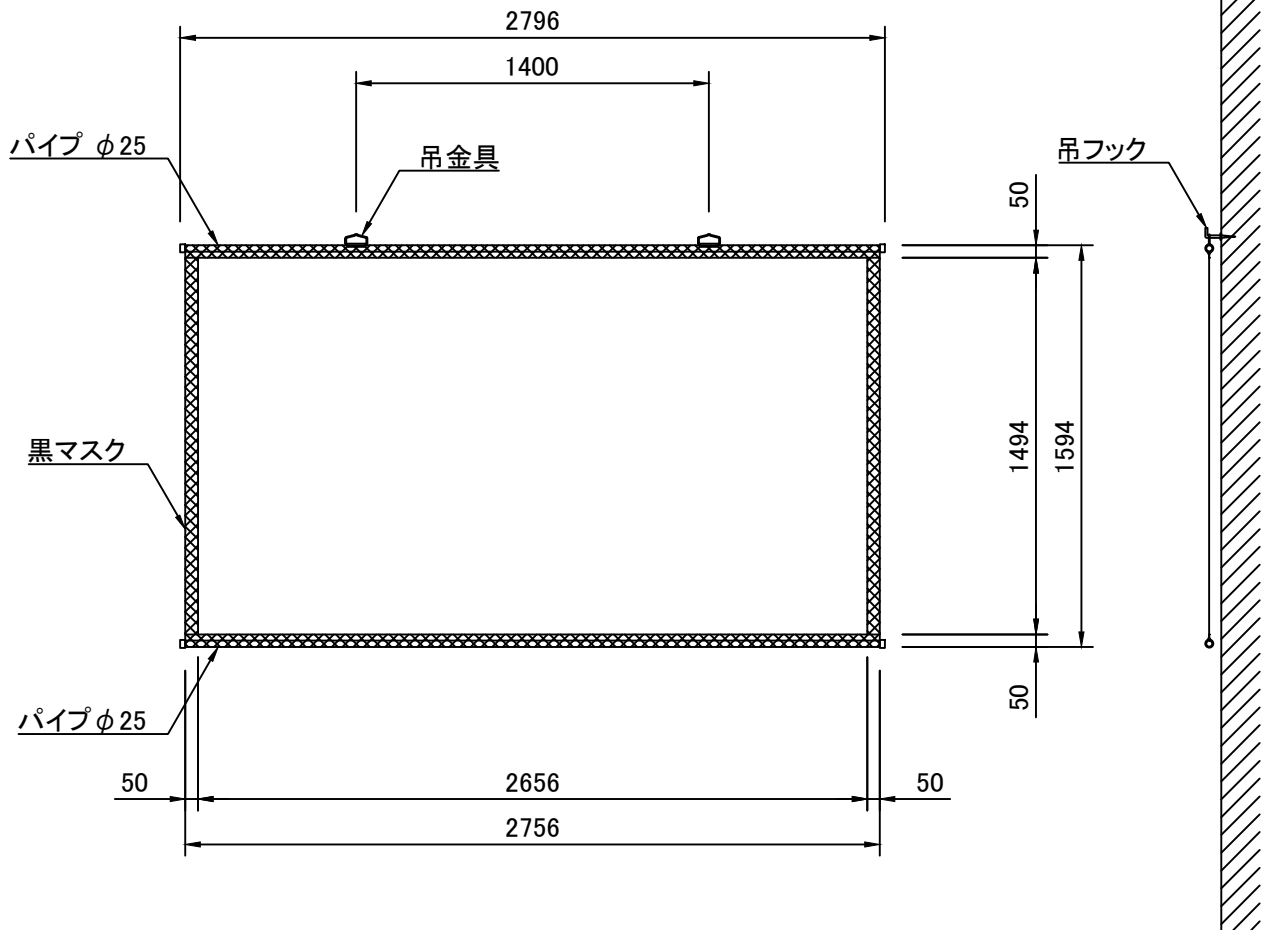
外観図 S=1/30
