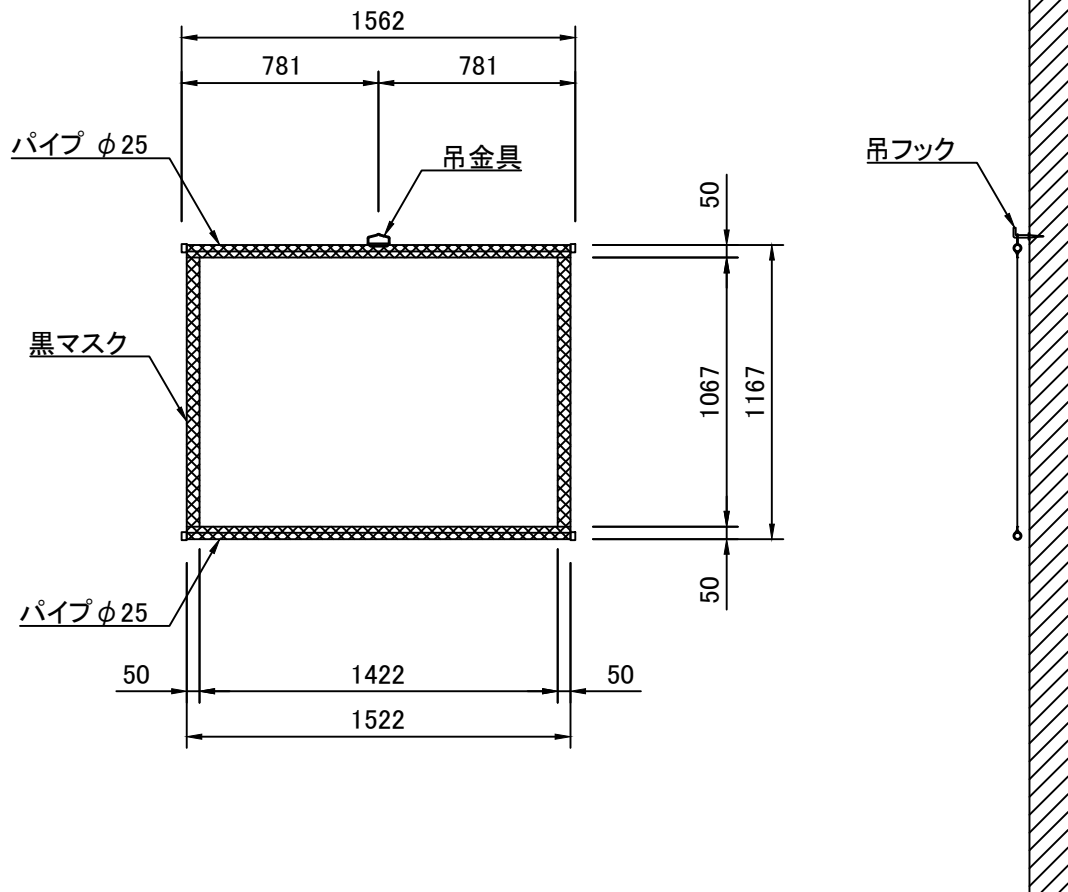
外観図 S=1/30
