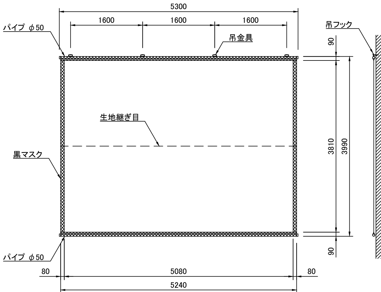
外観図 S=1/50
