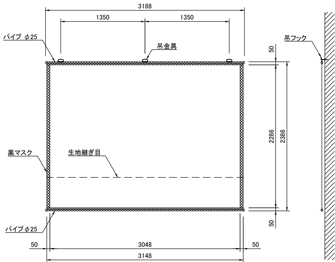
外観図 S=1/30
