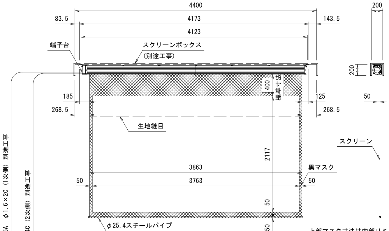
外觀図 S=1/40
