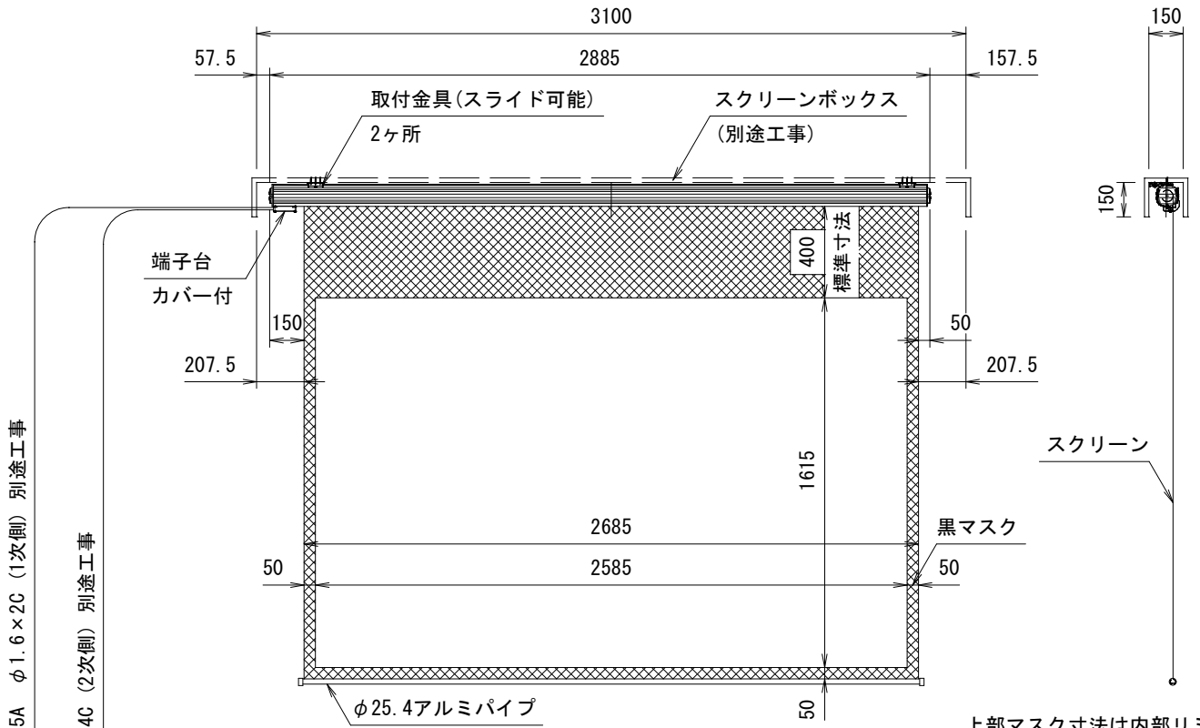
外觀図 S=1/30
