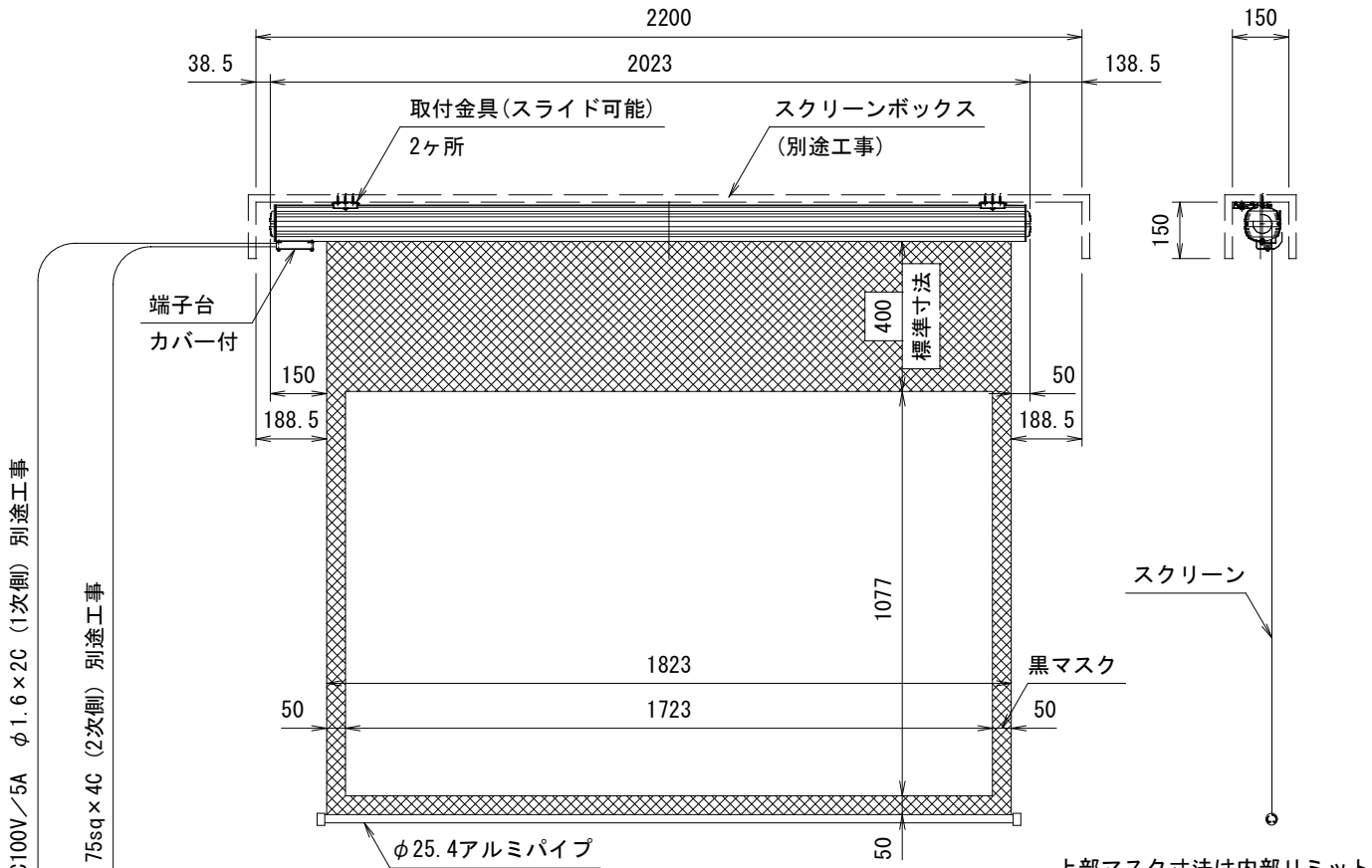
外觀図 S=1/20
