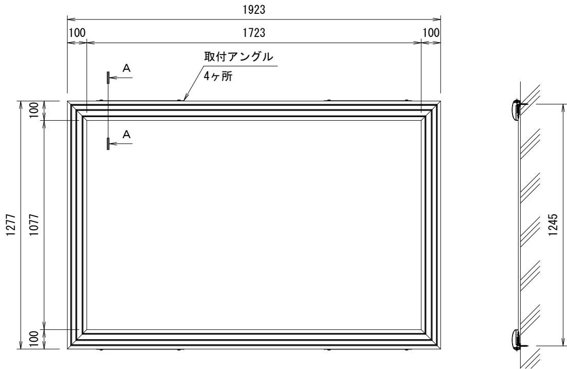
外観図 S=1/20
