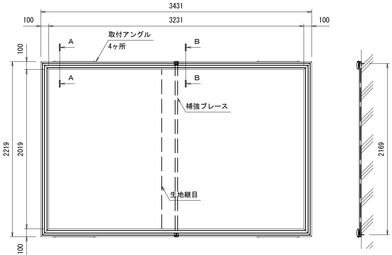
外観図 S=1/30
