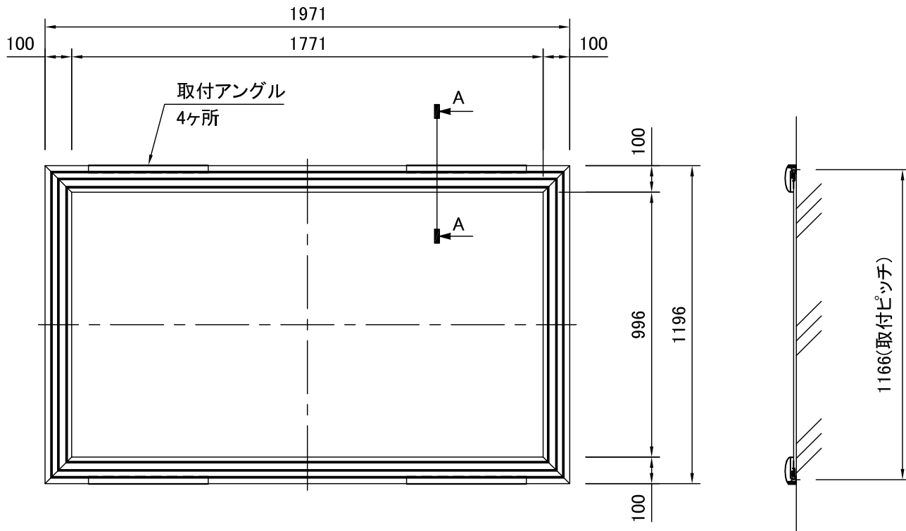
外観図 S=1/20
