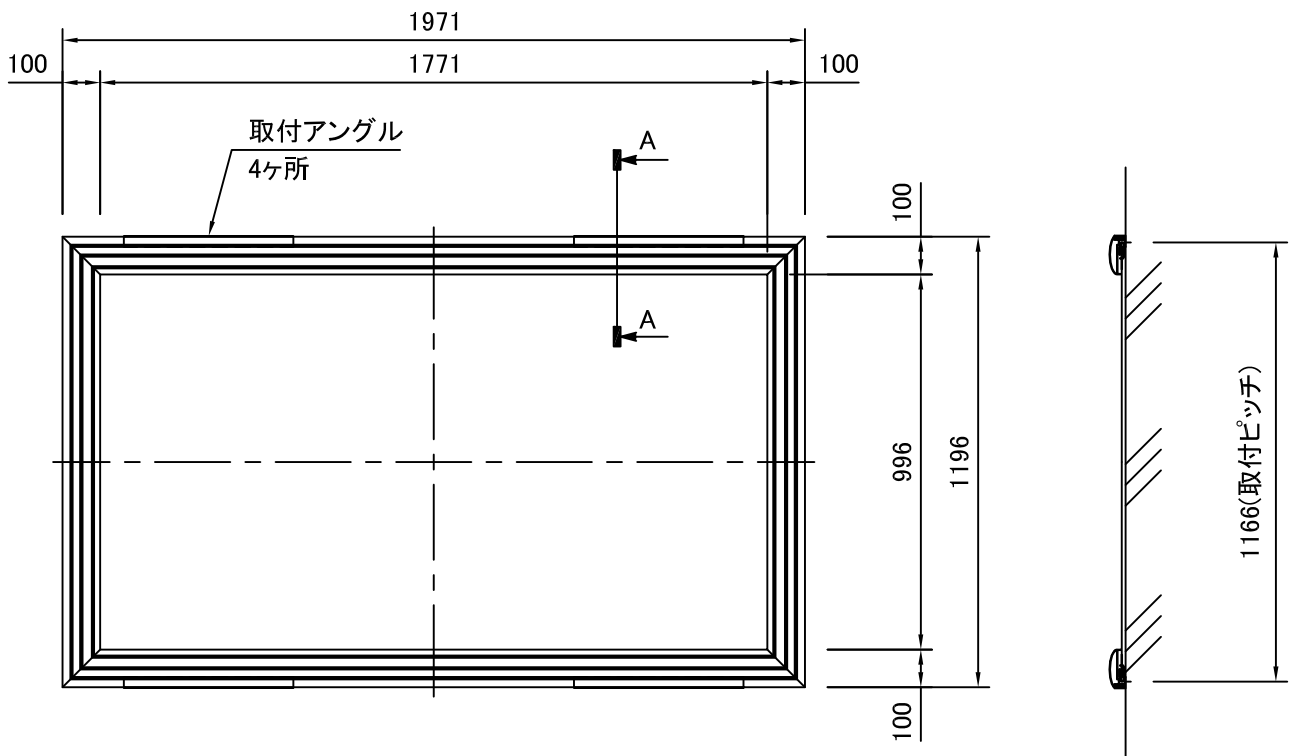
外観図 S=1/20
