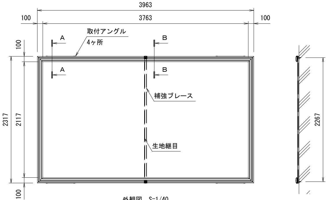
外観図 S=1/40
