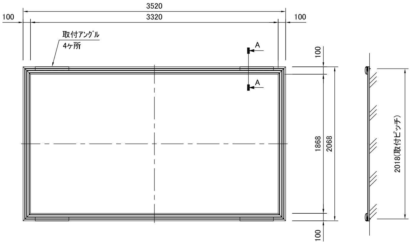
外觀図 S=1/30
