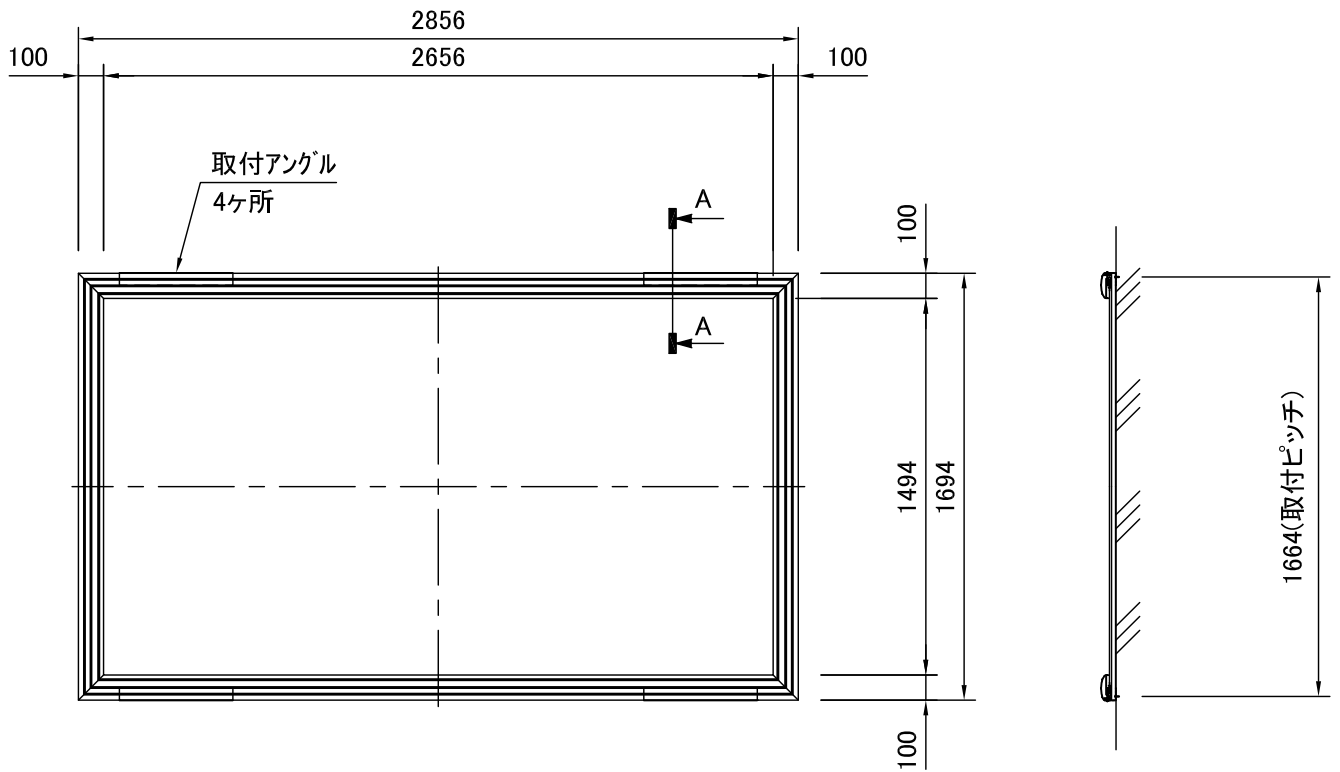
外観図 S=1/30
