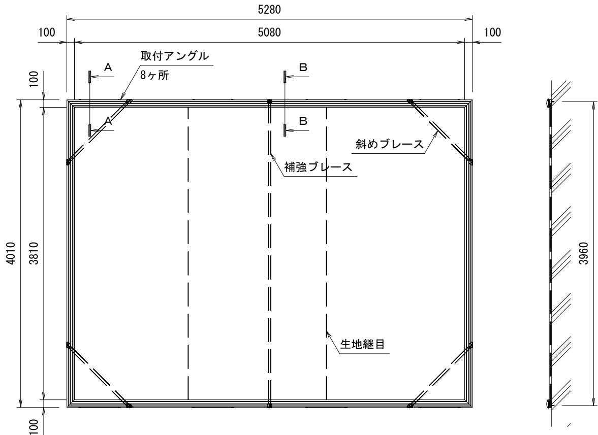
外觀図 S=1/50
