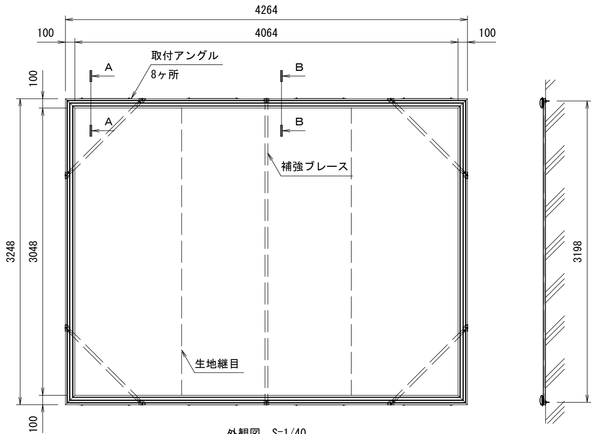
外観図 S=1/40
