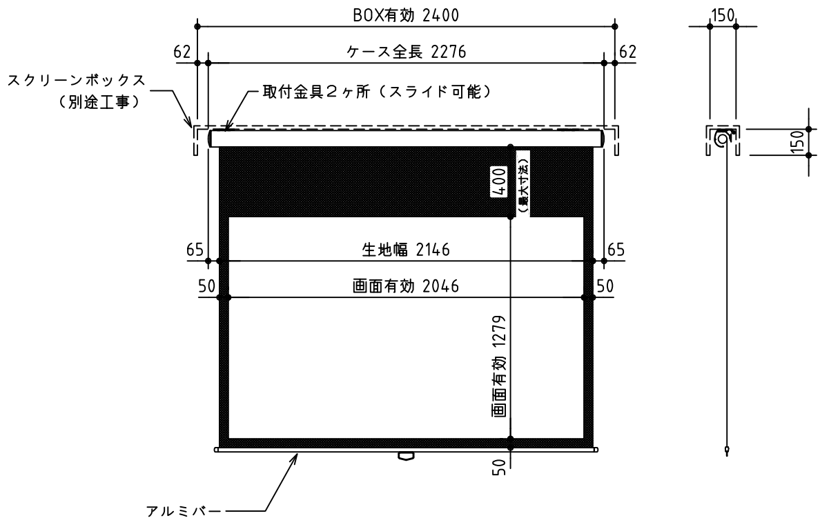
外観図 S=1/30
