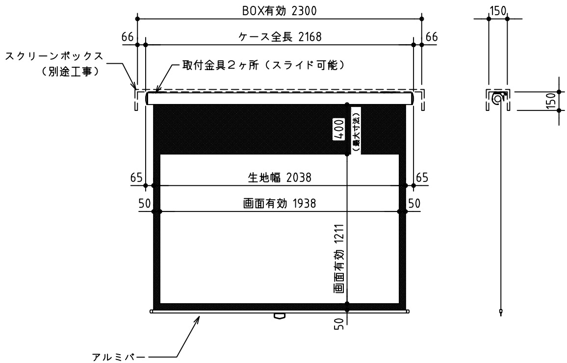
外觀図 S=1/30
