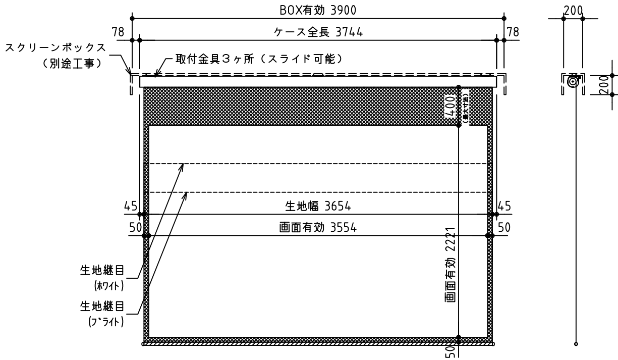
外觀図 S=1/40
