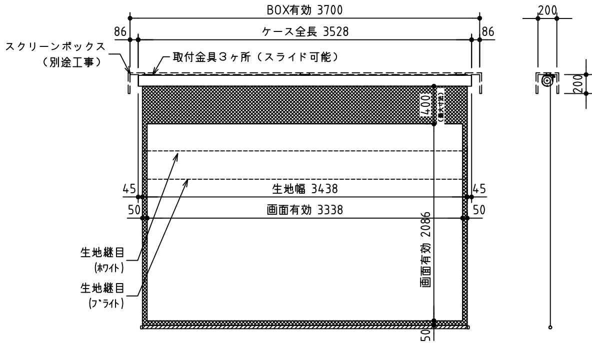
外観図 S=1/40
