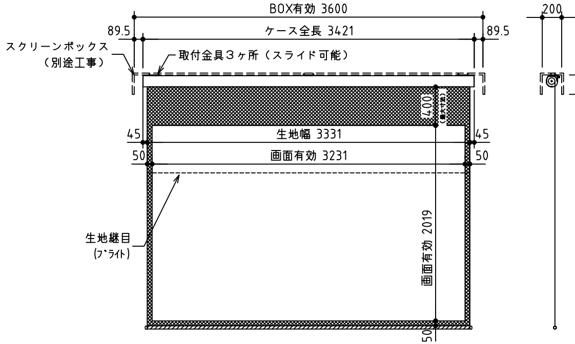
外観図 S=1/40
