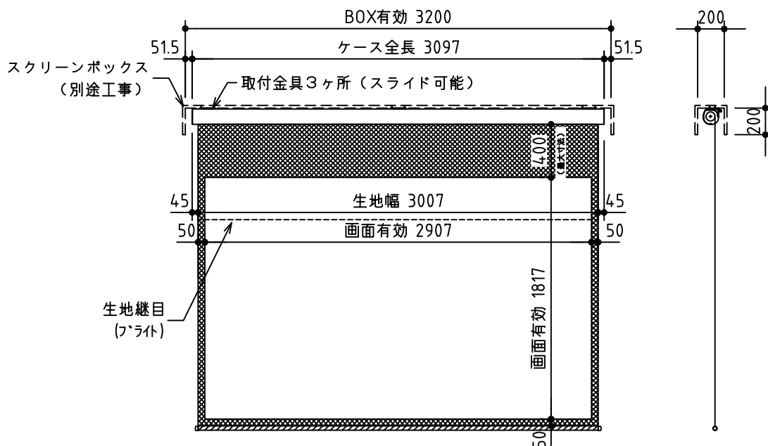
外觀図 S=1/40
