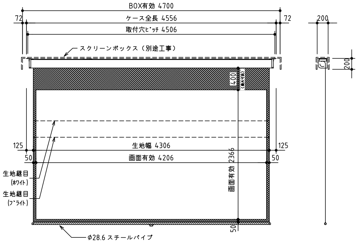
外觀図 S=1/40
