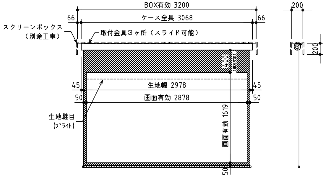
外観図 S=1/40
