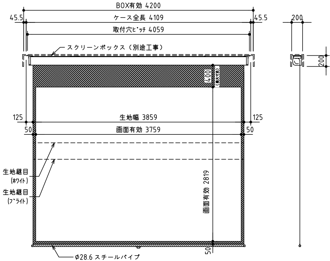
外觀図 S=1/40
