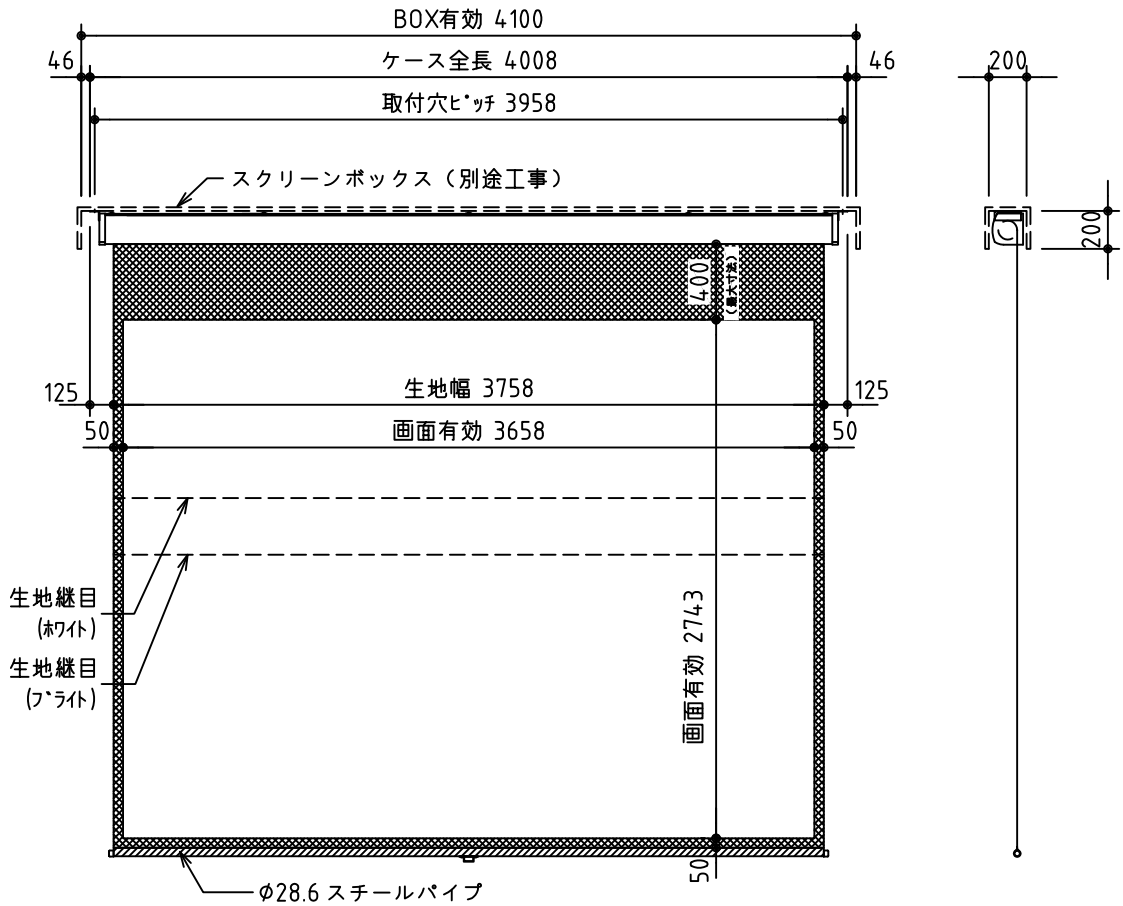
外觀図 S=1/40
