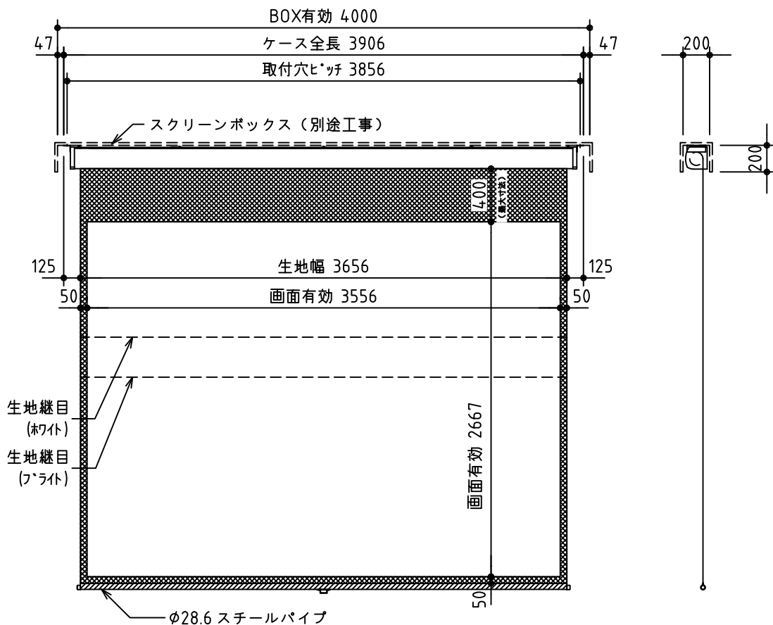
外觀図 S=1/40
