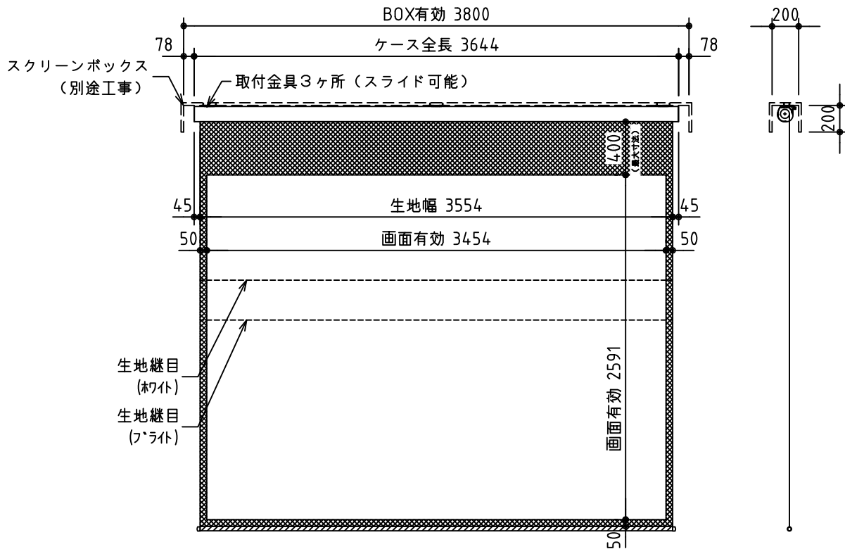
外観図 S=1/40
